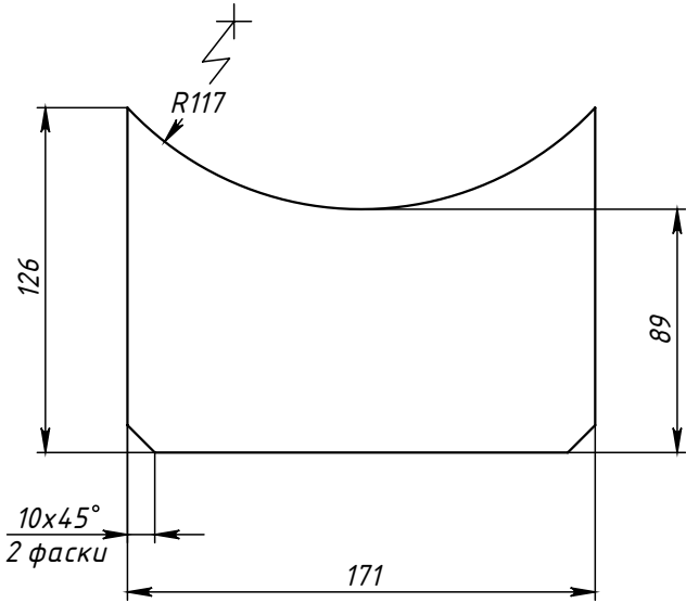
Поз.2 (Ребро)
