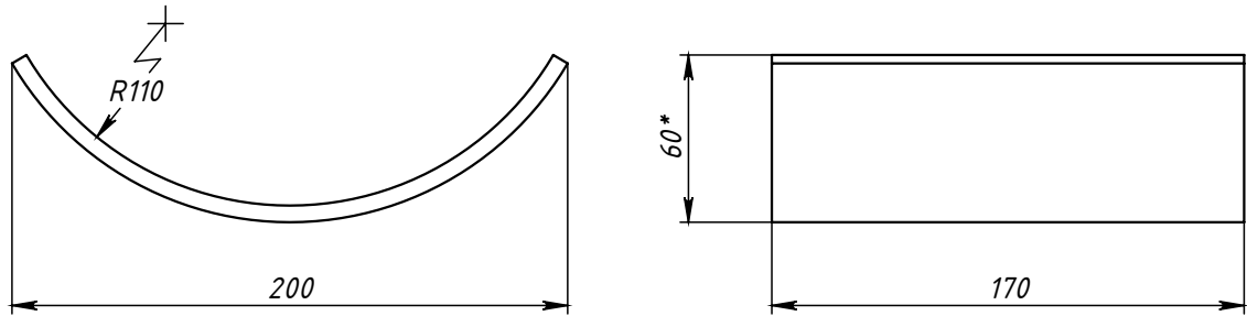
Поз.3 (Ложемент)
