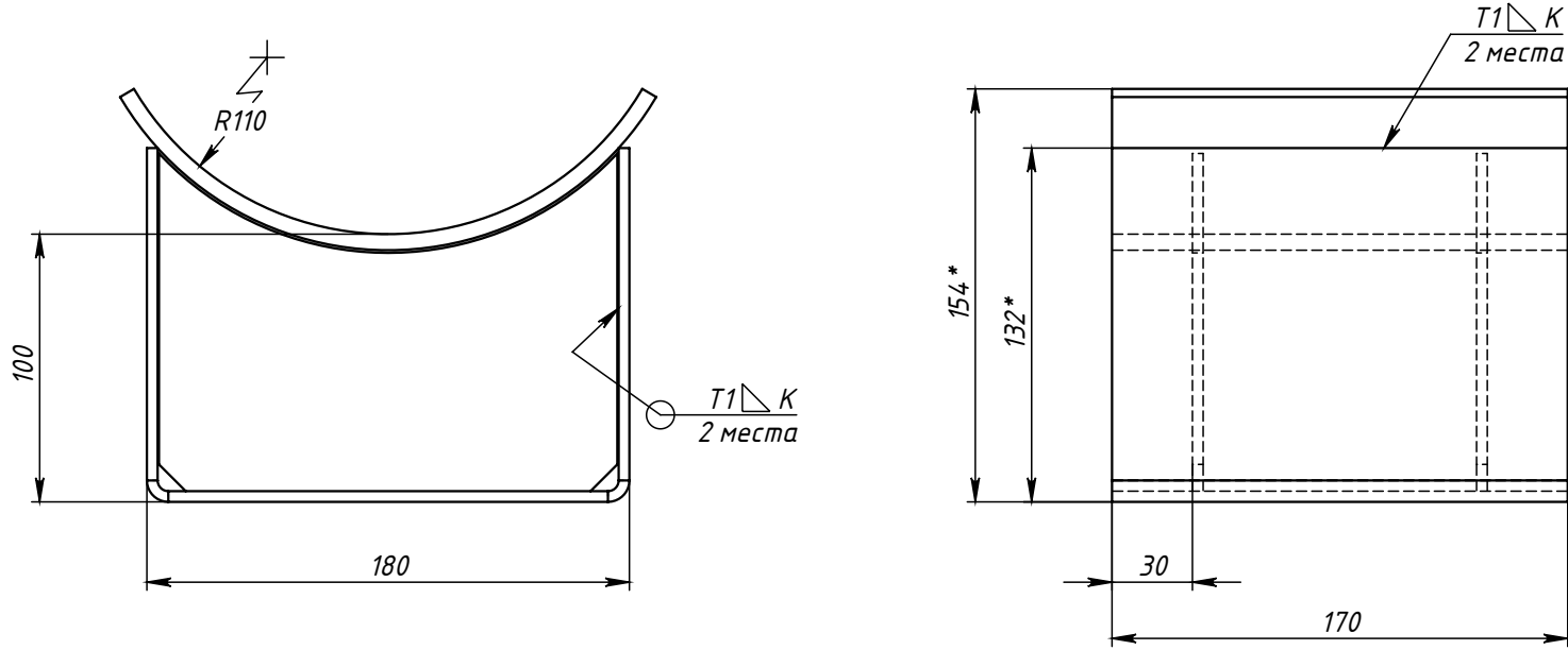
Поз.3 (Ложемент)
